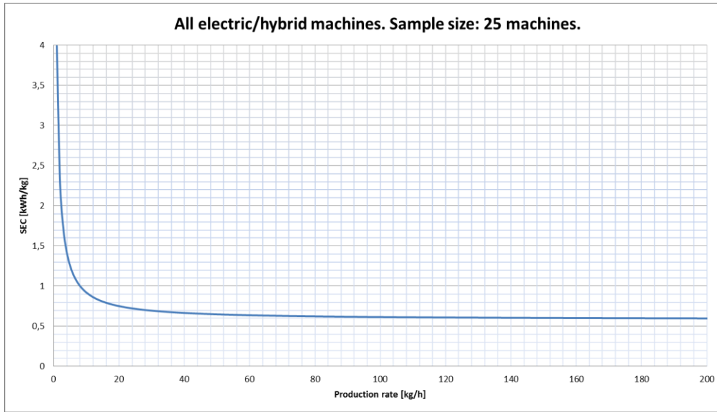
Figura 16: variazione del consumo specifico di riferimento delle presse elettriche e ibride in funzione del Production rate
