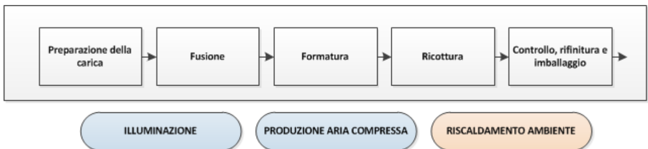
Figura 14: schema a blocchi del processo produttivo
