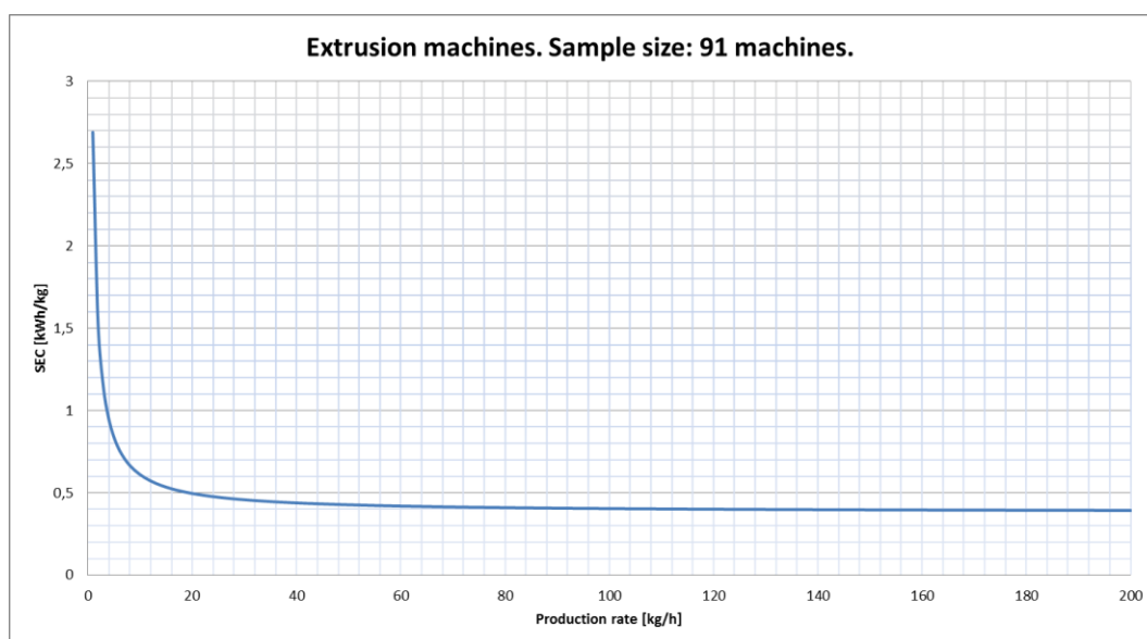
Figura 18: variazione del consumo specifico degli estrusori di profili e film in bolla in funzione del Production rate
